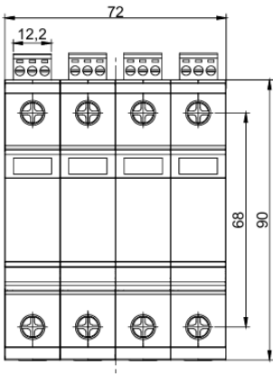
Габаритные размеры
