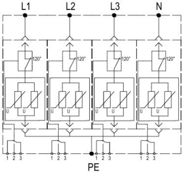
Принципиальная схема
